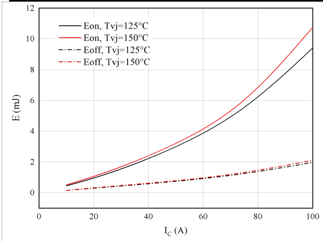
图 7. 开关损耗
