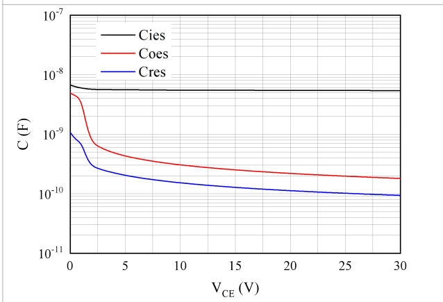
图 11. 电容特性
