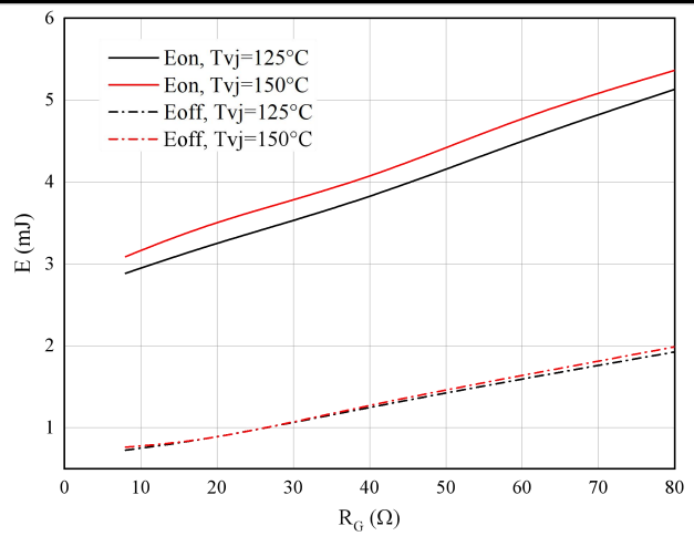
图 8. 开关损耗
